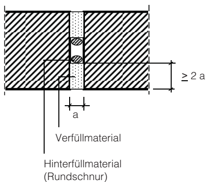
Abb. 2: Vertikalfuge nur im Randbereich verfüllt
