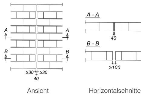
Abb. 3: Vertikalfuge mit Verzahnung
