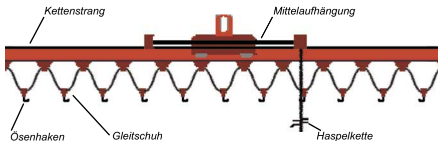
Bild 14: Ausschnitt Ausgleichstraverse (Beispielhafte Darstellung)
