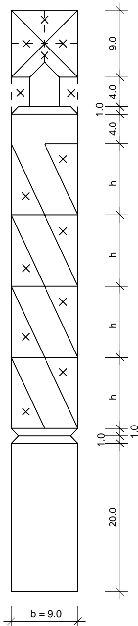
SEITENANSICHT
